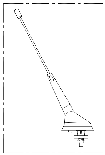
DET. VISTA EXPLODIDA ESC.: 1:3
