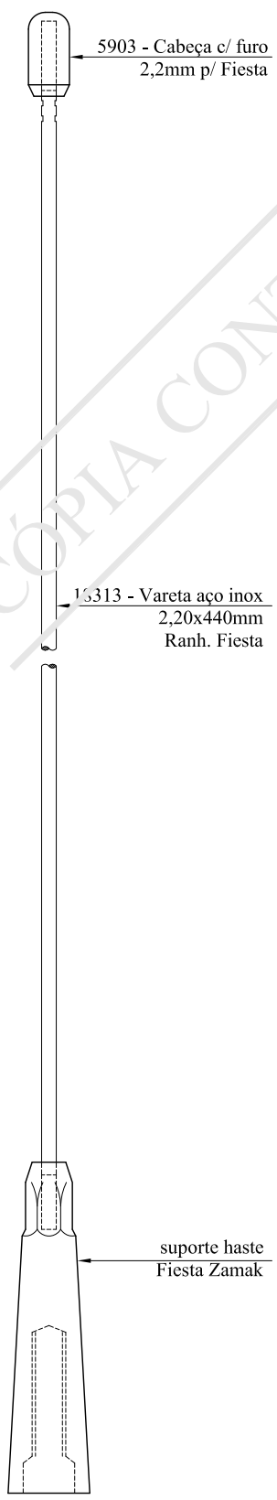
VISTA EXPLODIDA ESC.: 1:1
