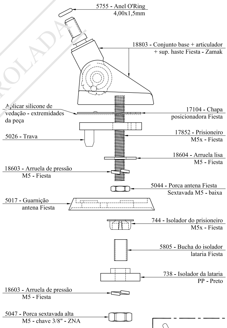
VISTA EXPLODIDA ESC.: 1:1
