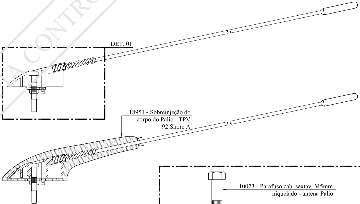
4050 - Subconjunto antena do Palio ESC.: 1:2
