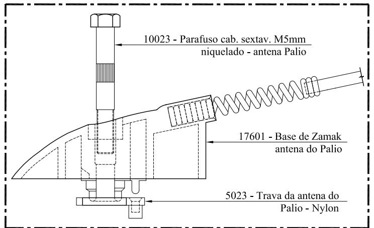
DETALHE 01 ESC.: 1:1
