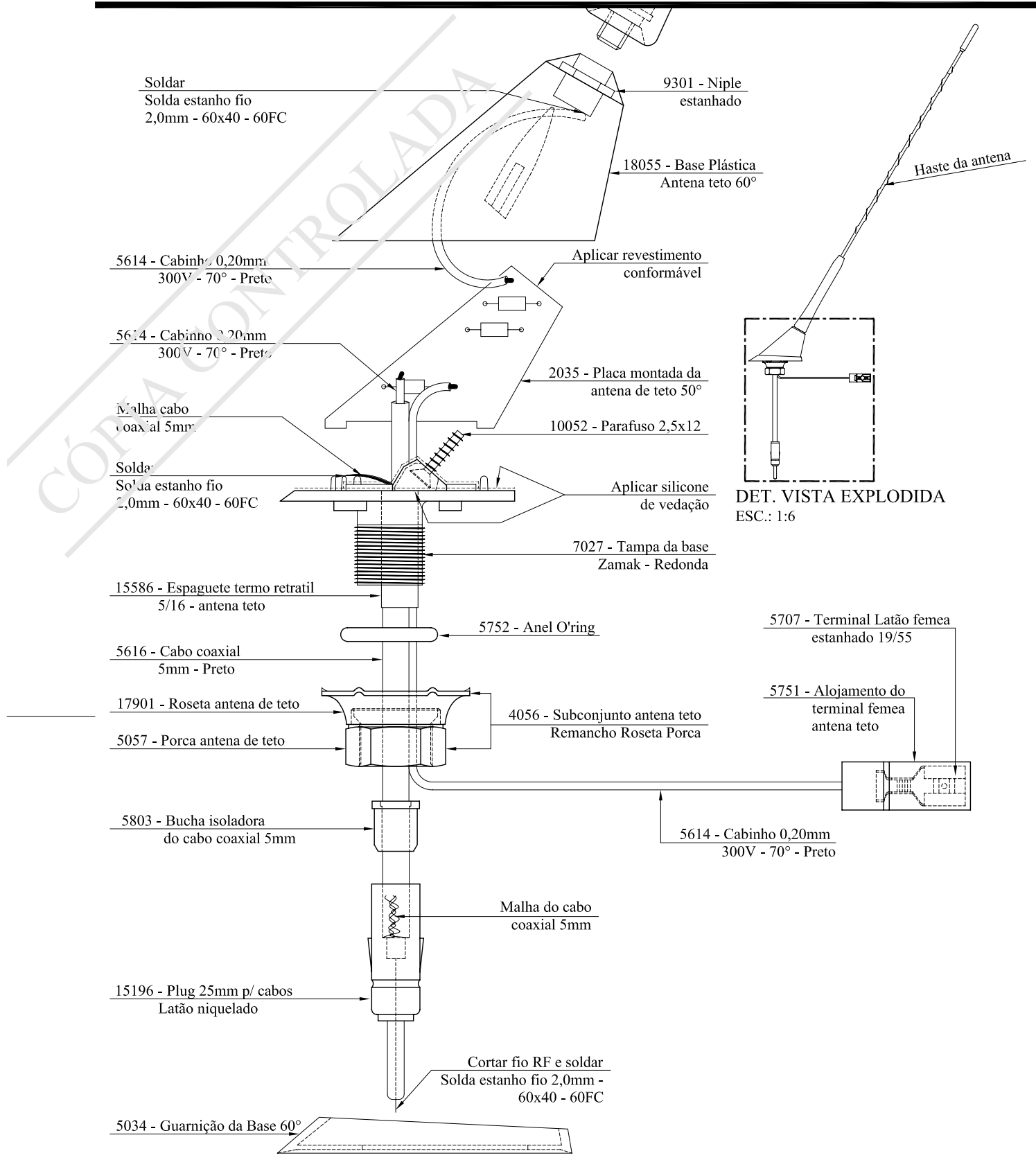
VISTA EXPLODIDA ESC.: 1:1
