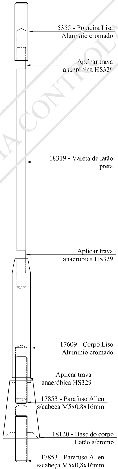
VISTA EXPLODIDA 3901 - Subconjunto Mini Haste Lisa Aluminiu VR/PT
