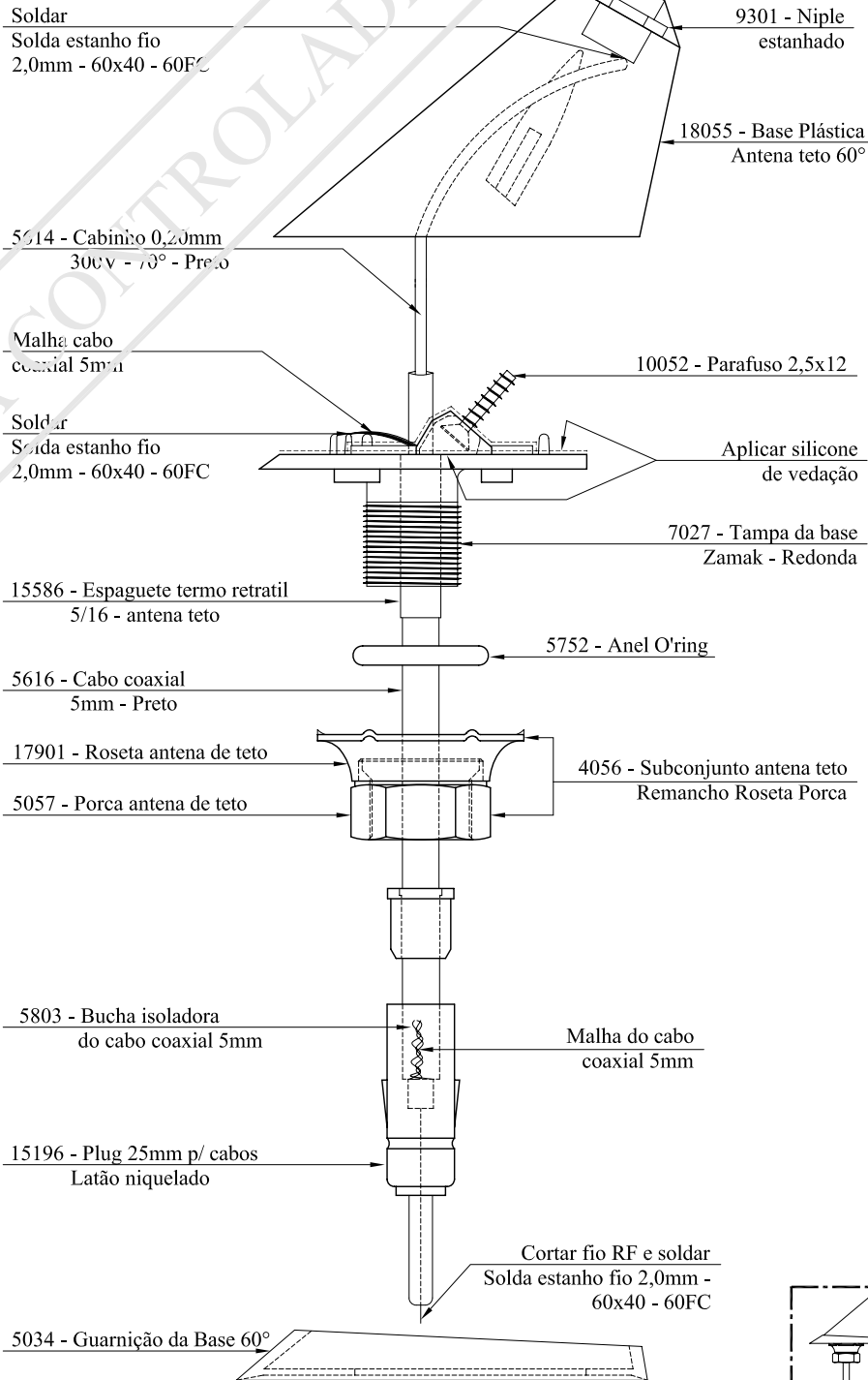
VISTA EXPLODIDA ESC.: 1:1
