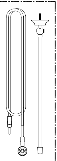
DET. VISTA EXPLODIDA ESC.: 1:5
