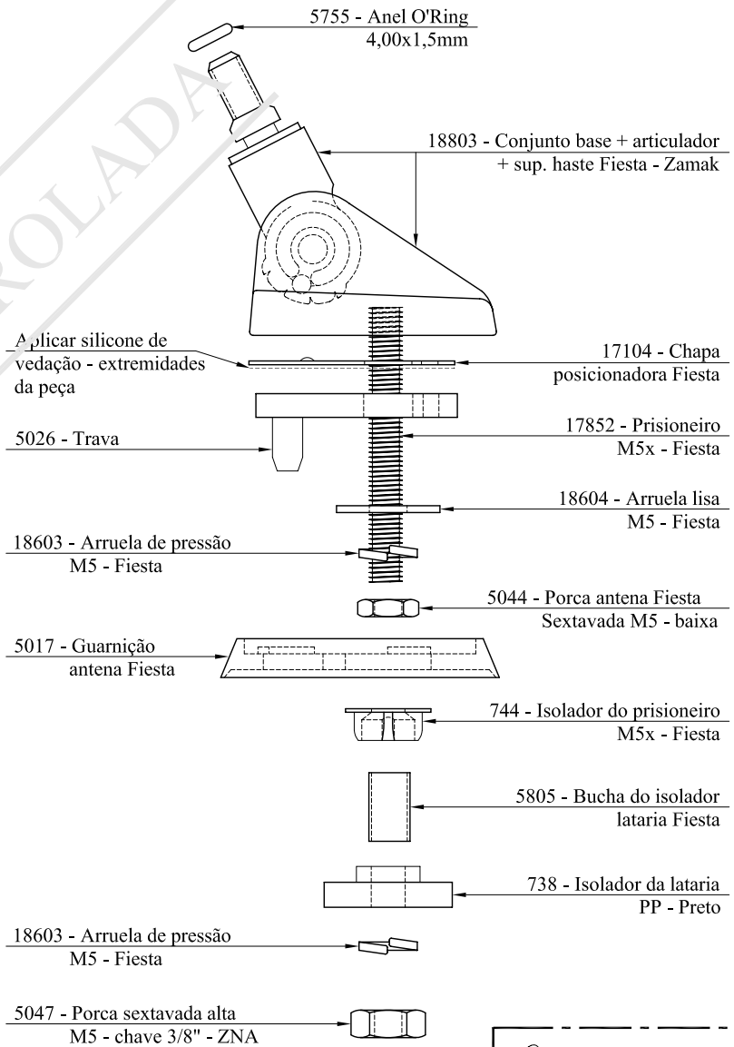
VISTA EXPLODIDA ESC.: 1:1
