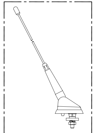
DET. VISTA EXPLODIDA ESC.: 1:3
