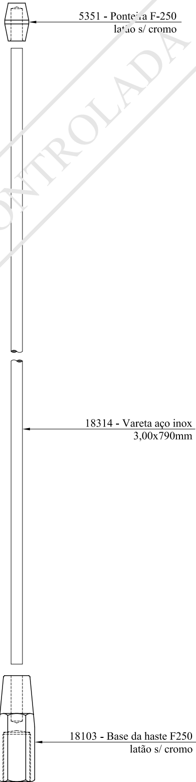
VISTA EXPLODIDA 4075 - Subconjunto F250 preta ESC.: 1:1
