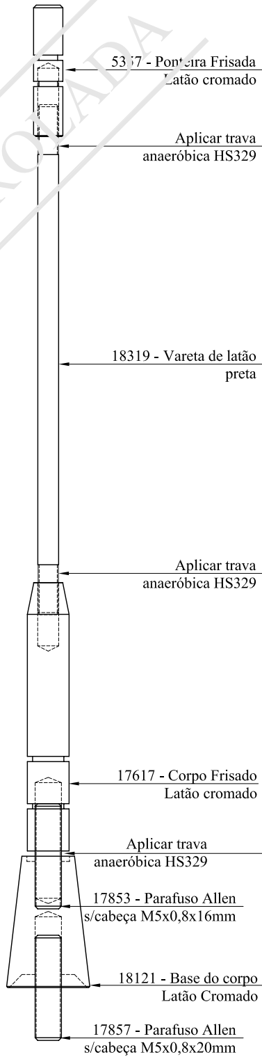
VISTA EXPLODIDA 4123 - Subconjunto Mini Haste Frisada Cromada Citroen
