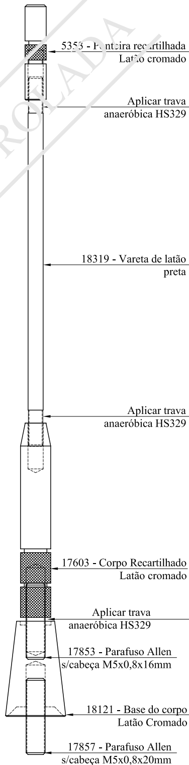
VISTA EXPLODIDA 4121 - Subconjunto Mini Haste Recartilhada Cromada Citroen
